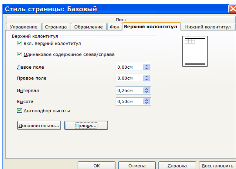
Рисунок 7 – Создание колонтитулов
